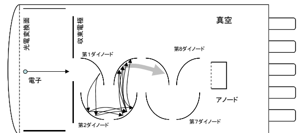
Fig. 18 光電子増倍管の概略図（ヘッドオン型）
