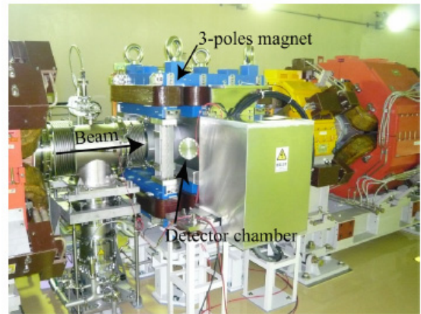
Fig. 10 RCS用水平タイプ IPMの概観
